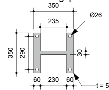
Forankringsplade 1:20
