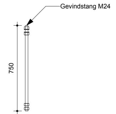
Gevindstang 1:20
