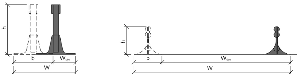
Figur 7.41 Princip for trafikværns arbejdsbredde W og udbøjningsbredde W_{dyn} .
